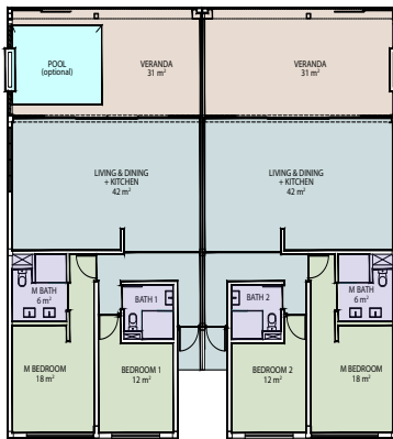
Ground floor plan - 2 bedroom option Plan du rez-de chaussée - Appartement de 2 chambres à coucher
