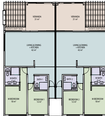
First floor plan - 2 bedroom option Plan du premier étage - Appartement de 2 chambres à coucher
