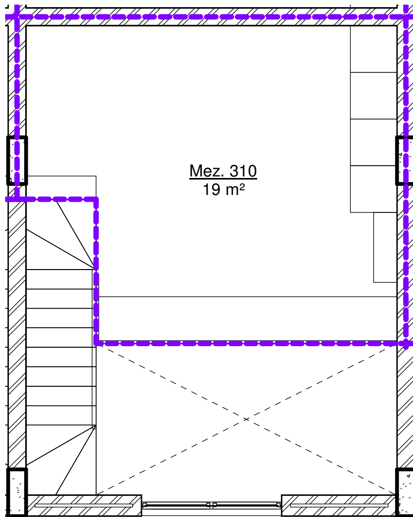
2 Unit 310 Upper Level 1 : 50
