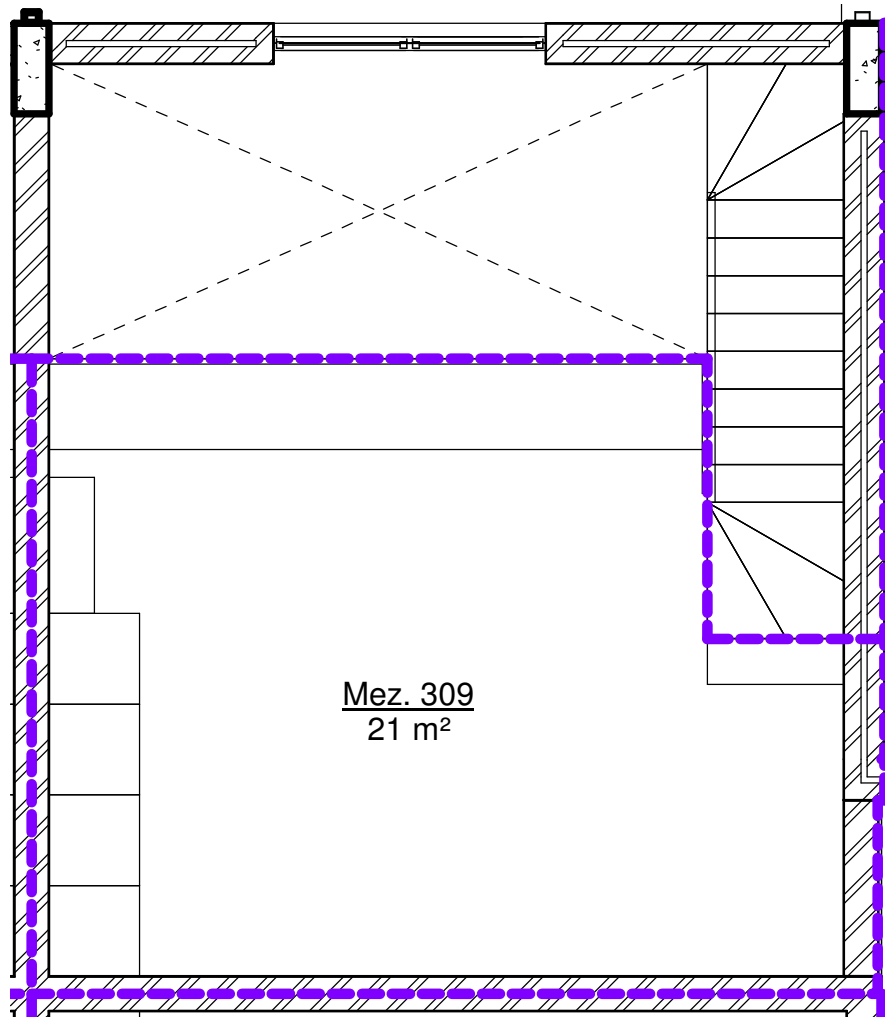
2 Unit 309 Upper Level 1 : 50
