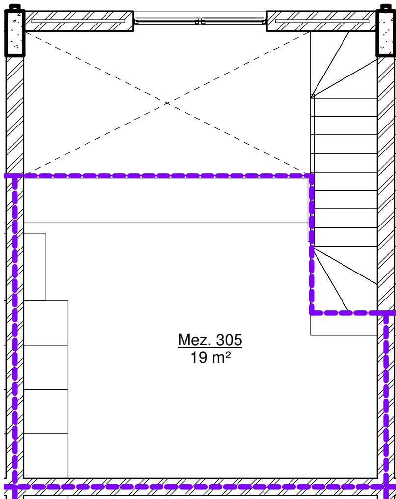
2 Unit 305 Upper Level 1 : 50
