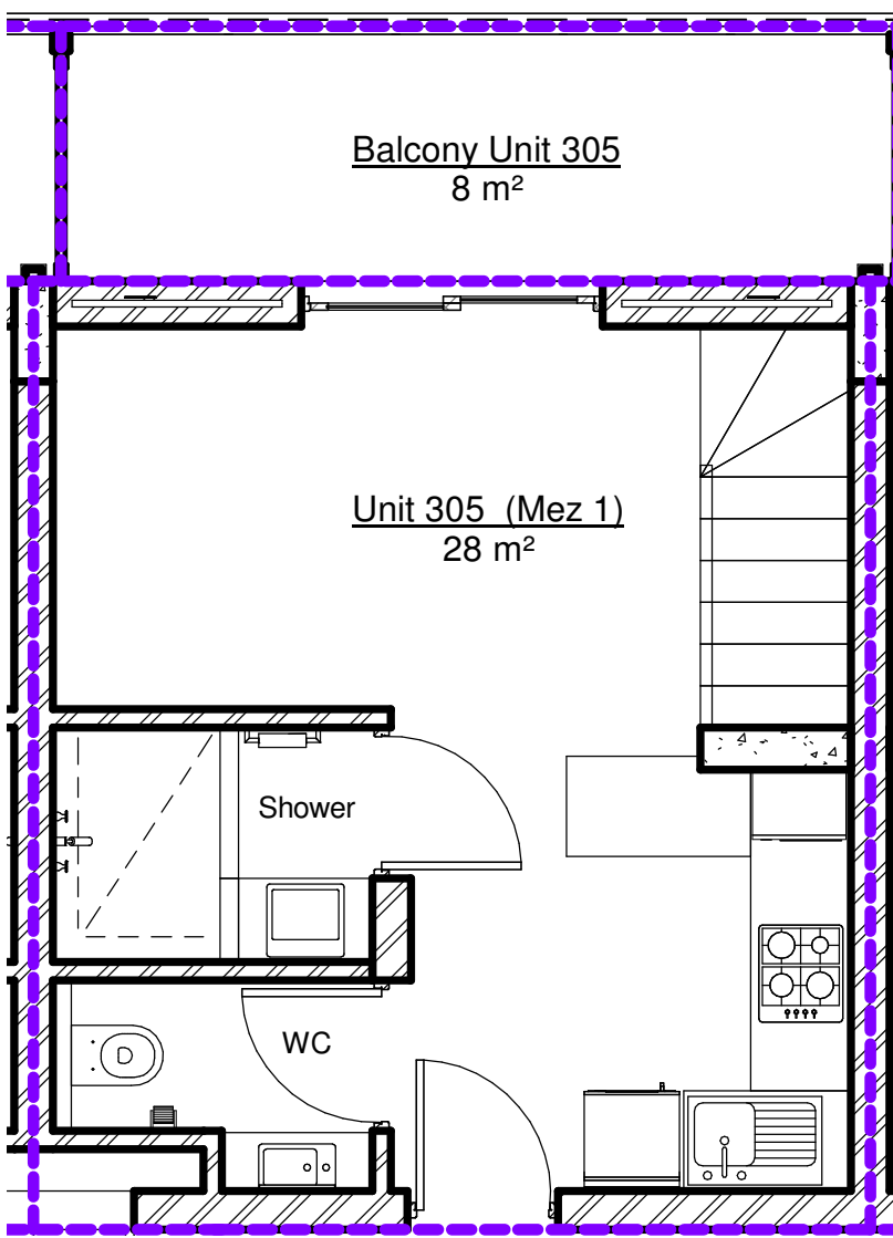
1 Unit 305 Lower Level 1 : 50
