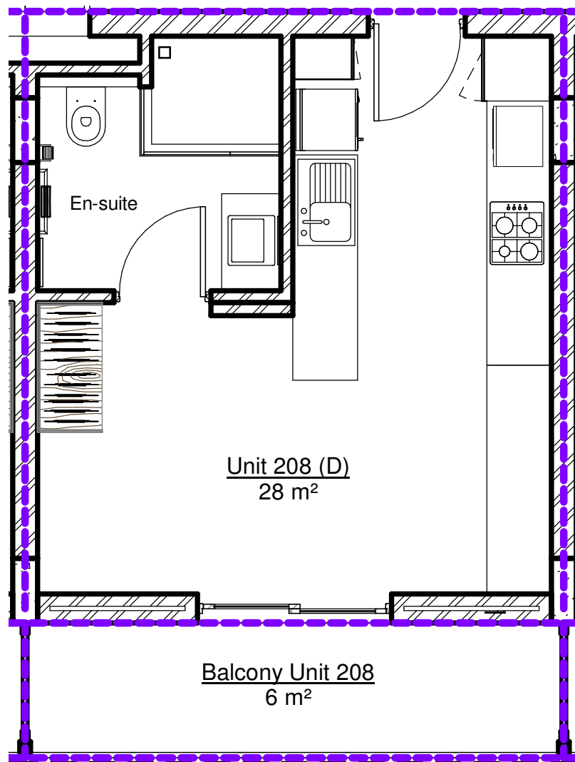
1 Unit 208 1 : 50
