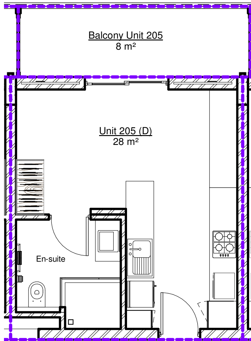
1 Unit 205 1 : 50
