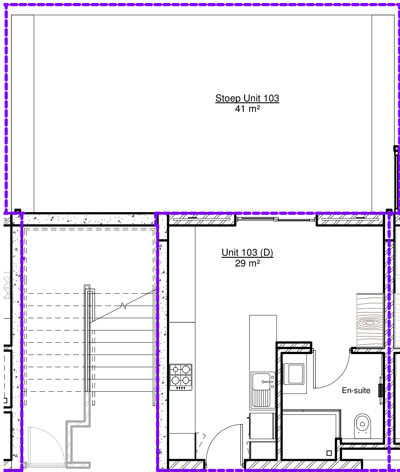
1 Unit 103 1 : 50
